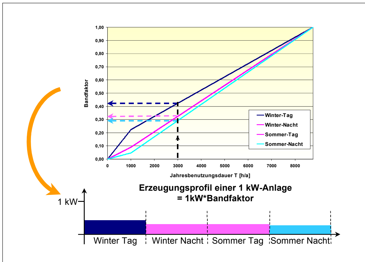
Bild 2: Beispiel für ein synthetisches Erzeugungsprofil für kleine KWK-Anlagen (< 30 kW)
