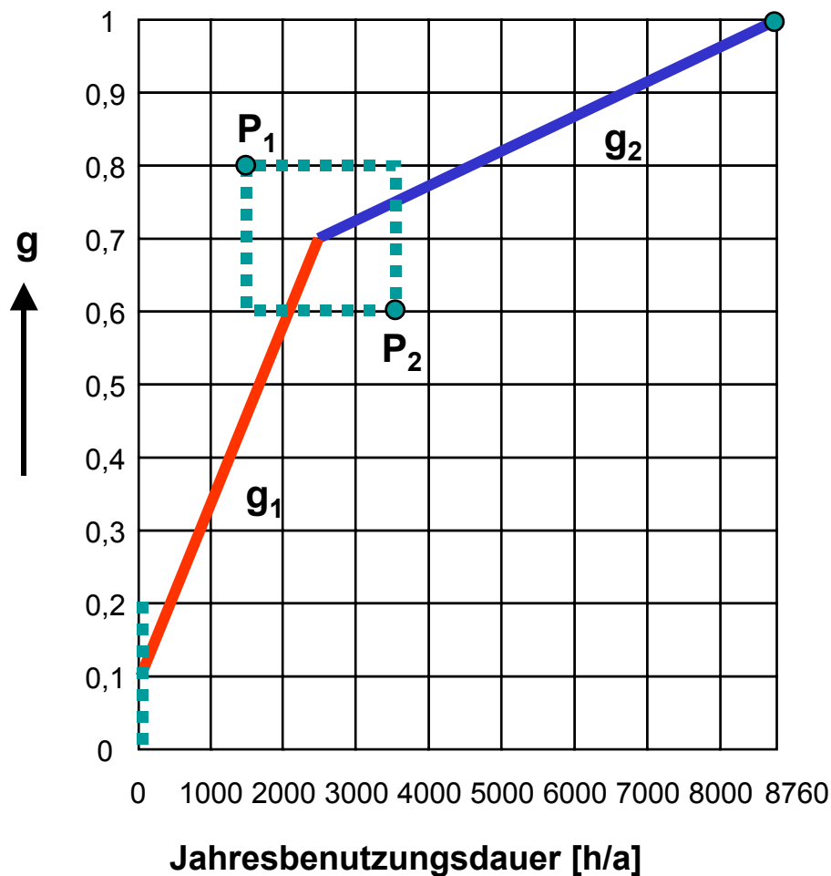
Abb. 1: Gleichzeitigkeitsgrad (Beispiel)
