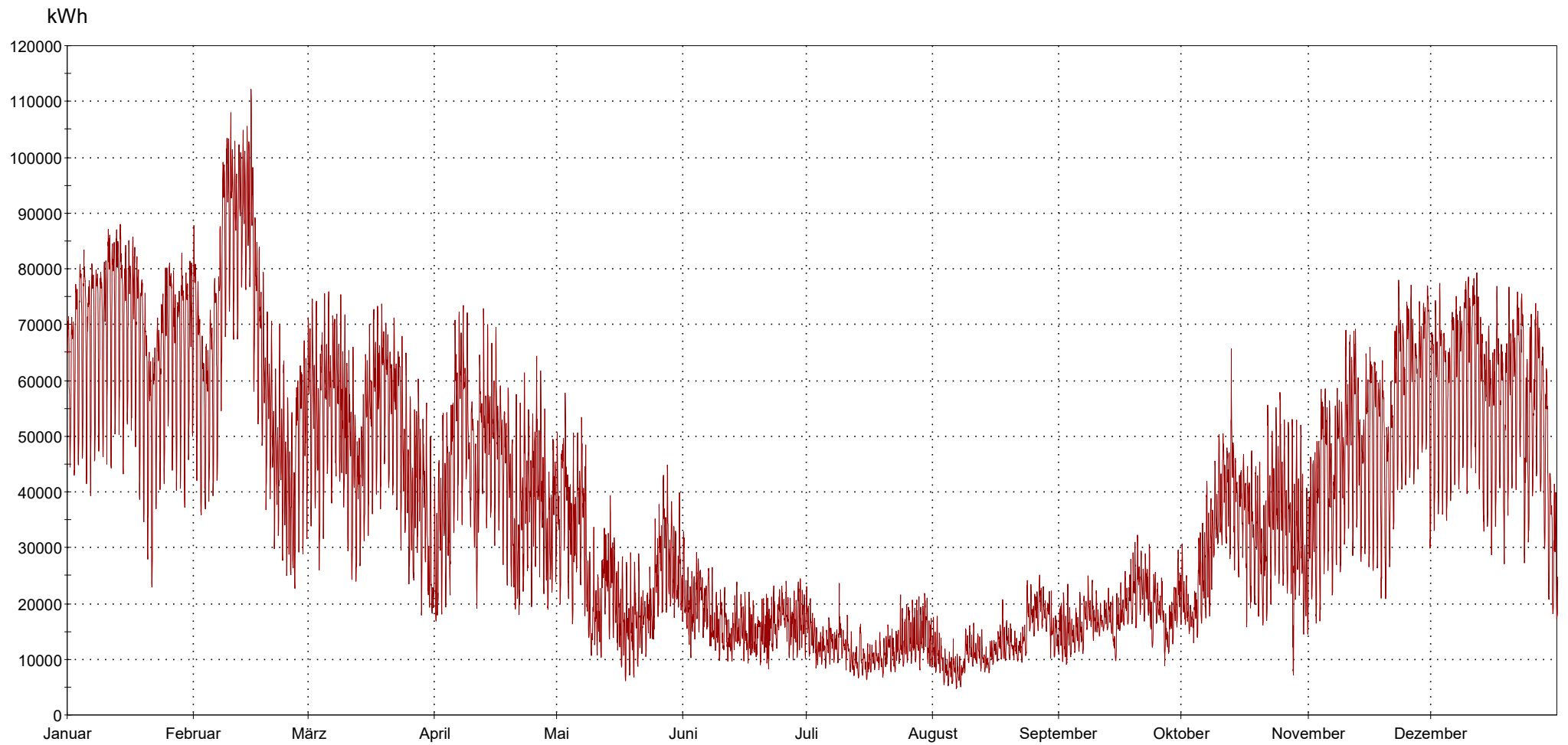
Jahreshöchstlast 112.194 kW - Lastverlauf als stündliche Leistungsmessung (Maximum am 15.02.2021 07:00 Uhr)
