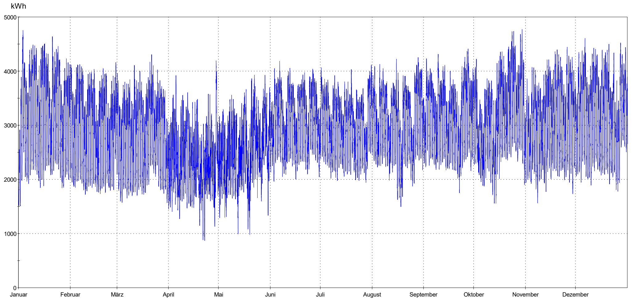
Jahreshöchstlast 19.089 kW - Lastverlauf viertelstündliche Leistungsmessung (Maximum am 29.10.2019 17:45 Uhr)
