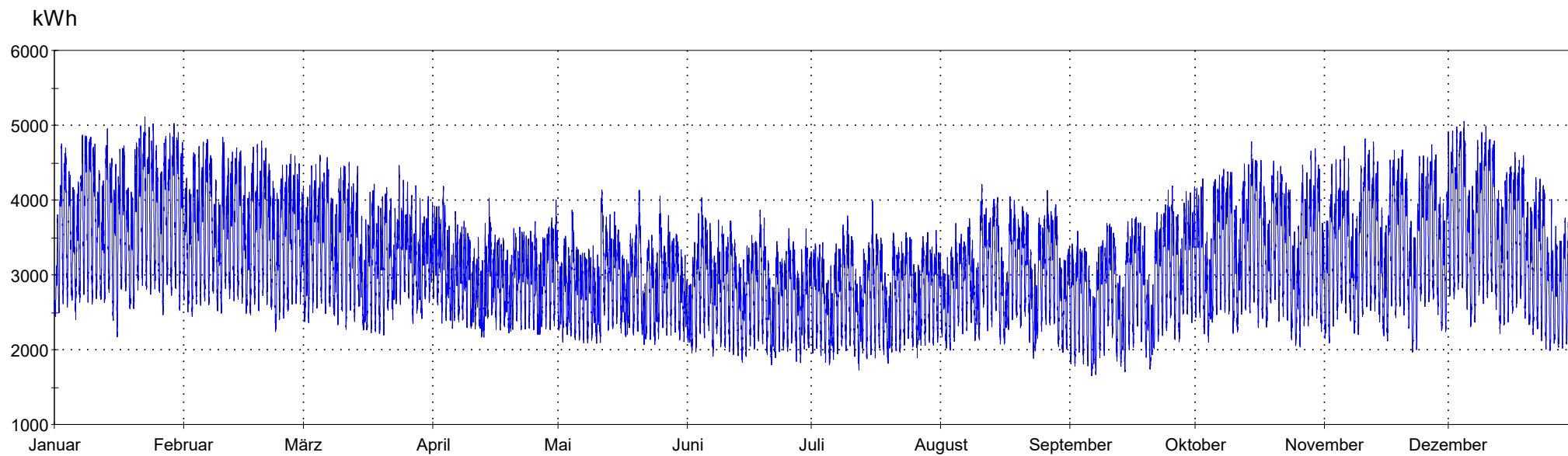
Jahreshöchstlast 20.447 kW - Lastverlauf viertelstündliche Leistungsmessung (Maximum am 22.01.2020 18:00 Uhr)
