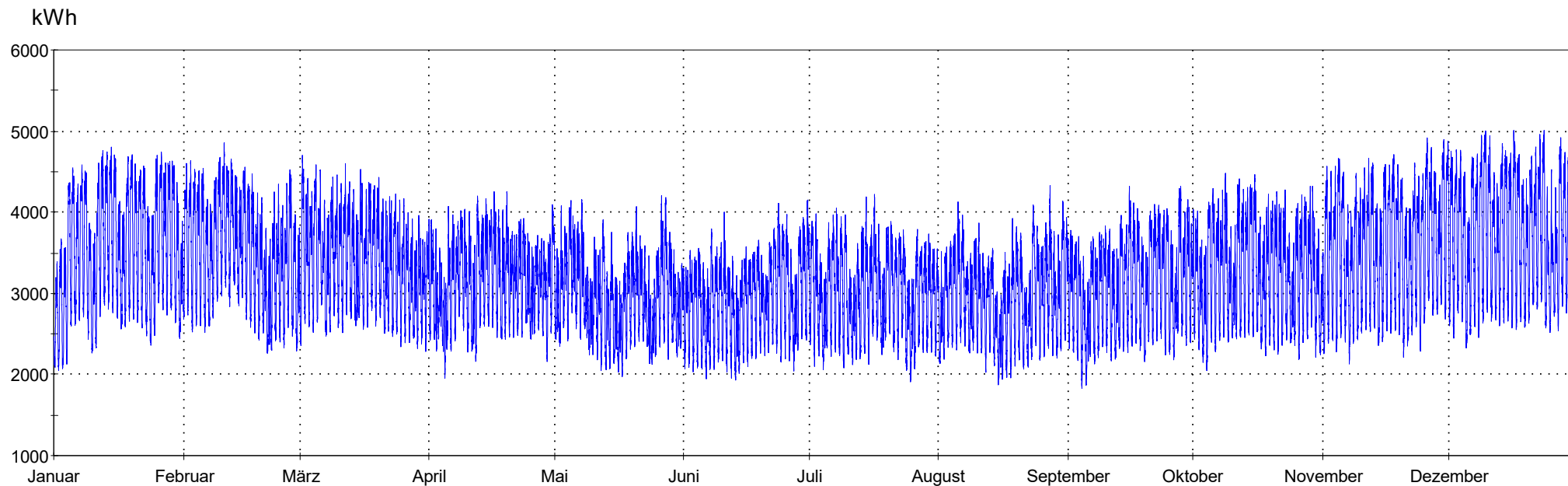
Jahreshöchstlast 20.045 kW - Lastverlauf viertelstündliche Leistungsmessung (Maximum am 16.12.2021 11:15 Uhr)
