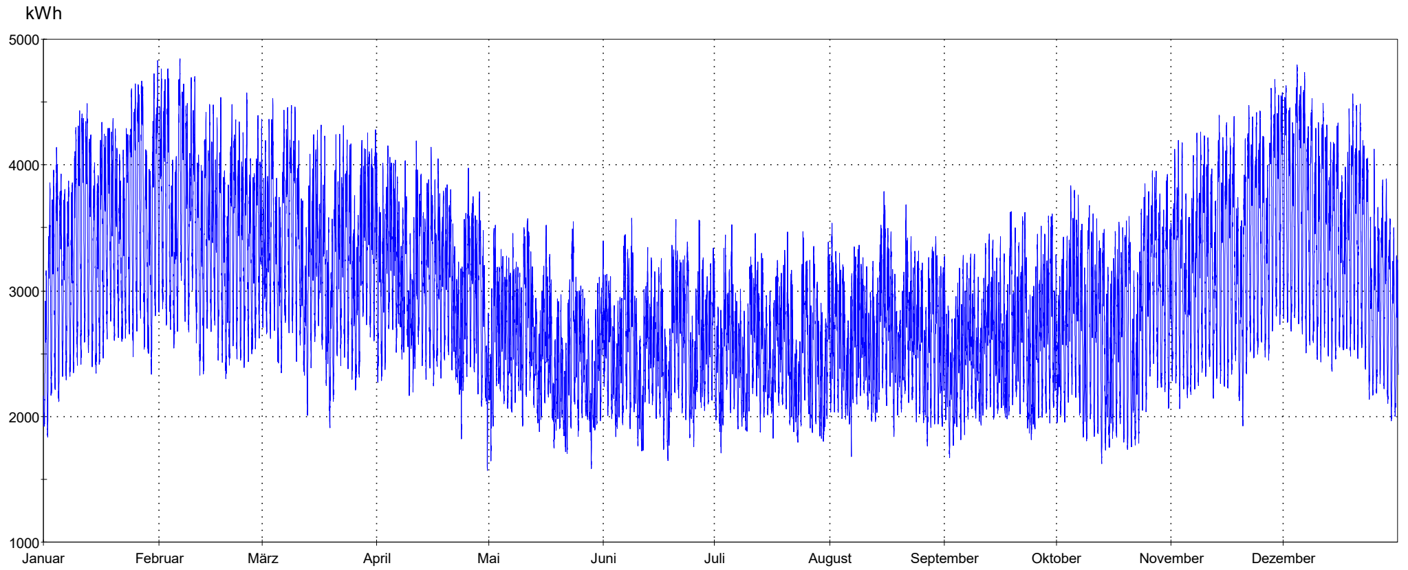
Jahreshöchstlast 19.377 kW - Lastverlauf viertelstündliche Leistungsmessung (Maximum am 06.02.2023 18:00 Uhr)
