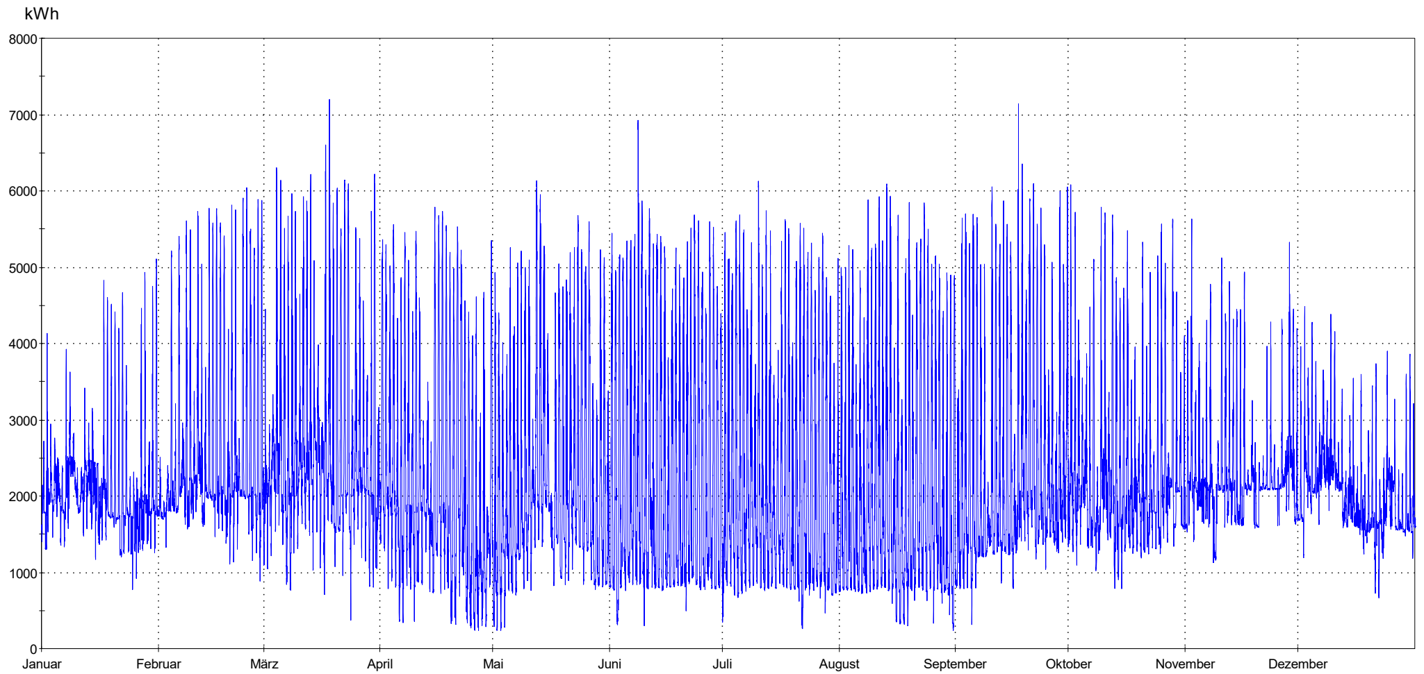
Summe aller Einspeisungen in die Mittelspannungsebene 78.592.456 kWh mit zeitlichem Verlauf
