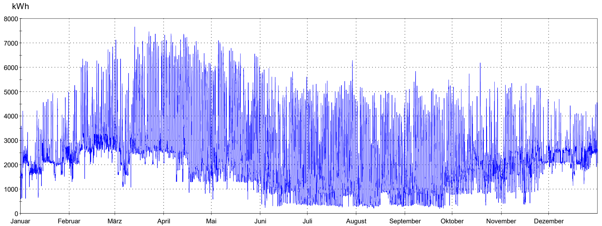
Summe aller Einspeisungen in die Mittelspannungsebene 81.730.042 kWh mit zeitlichem Verlauf
