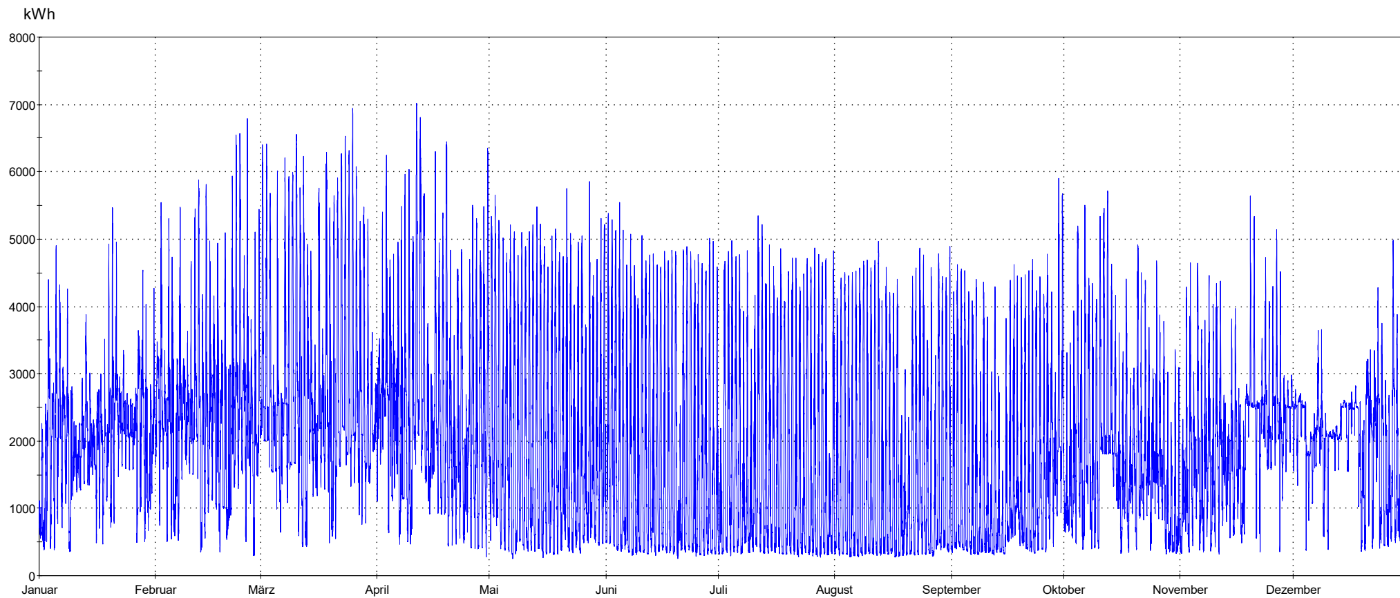
Summe aller Einspeisungen in die Mittelspannungsebene 69.552.630 kWh mit zeitlichem Verlauf
