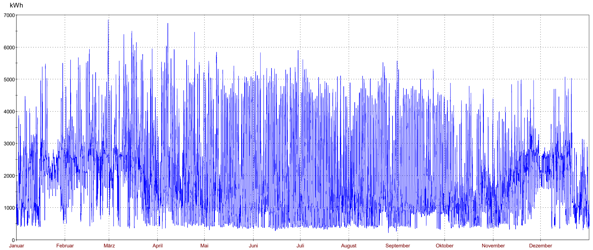
Summe aller Einspeisungen in die Mittelspannungsebene 67.430.133 kWh mit zeitlichem Verlauf
