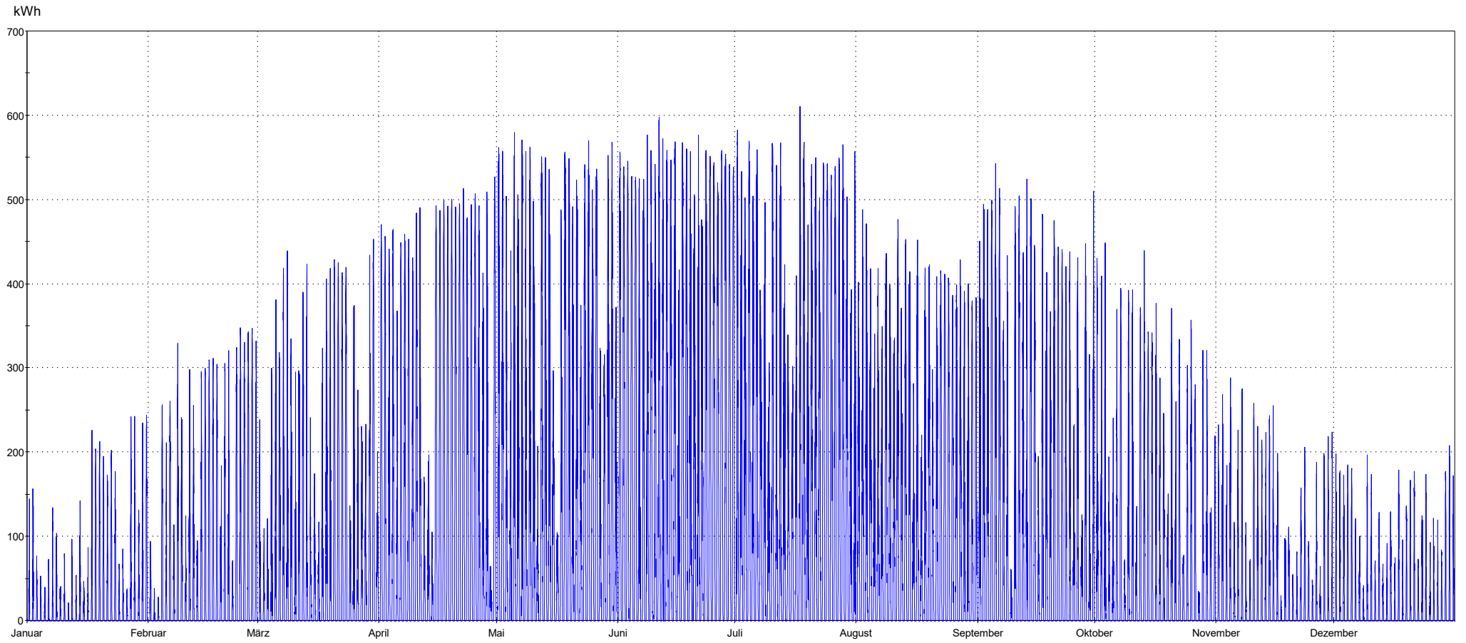
Summe aller Einspeisungen in die Niederspannungsebene 2.966.257 kWh mit zeitlichem Verlauf
