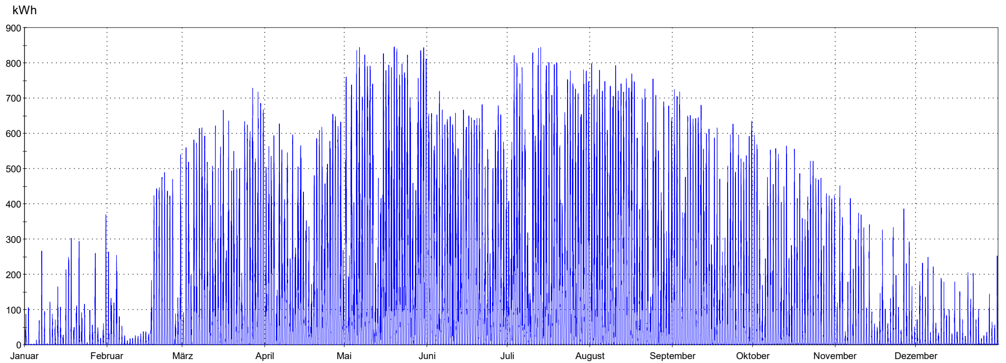
Summe aller Einspeisungen in die Niederspannungseben 3.726.170 kWh mit zeitlichem Verlauf
