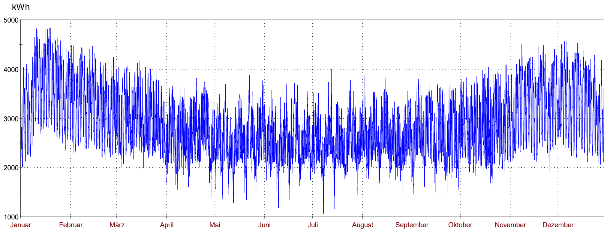
Jahreshöchstlast 19.418 kW - Lastverlauf viertelstündliche Leistungsmessung (Maximum am 18.01.2024 17:15 Uhr)
