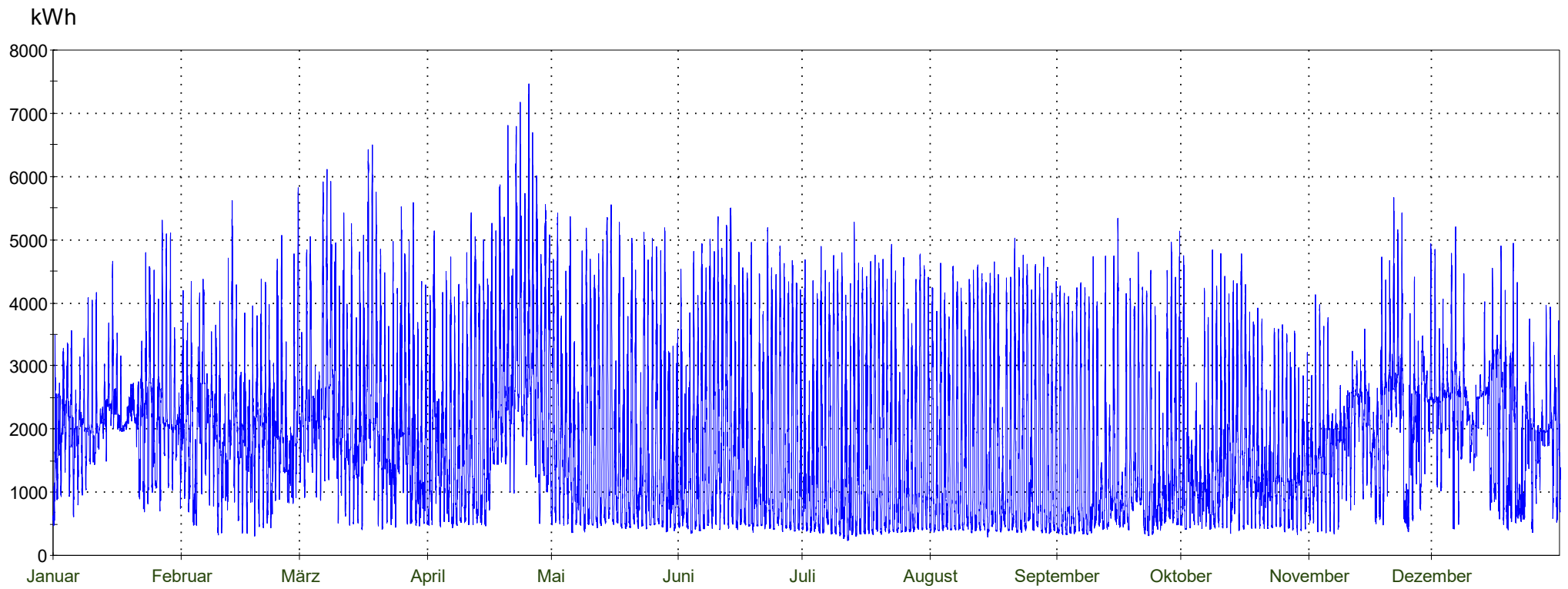
Summe aller Einspeisungen in die Mittelspannungsebene 65.593.553 kWh mit zeitlichem Verlauf
