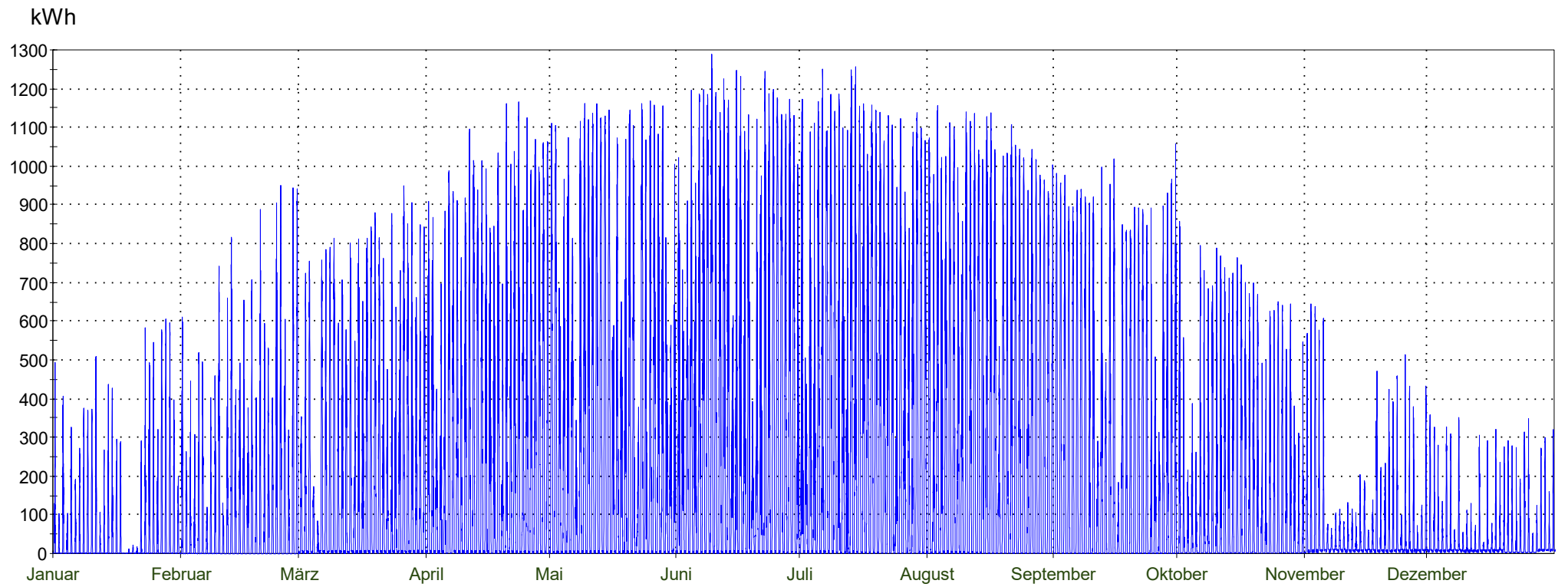
Summe aller Einspeisungen in die Niederspannungseben 6.237.503 kWh mit zeitlichem Verlauf
