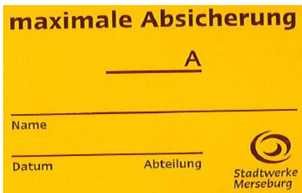
Abb. 4: Angabe der Nennstromstärke der HA-Sicherung
