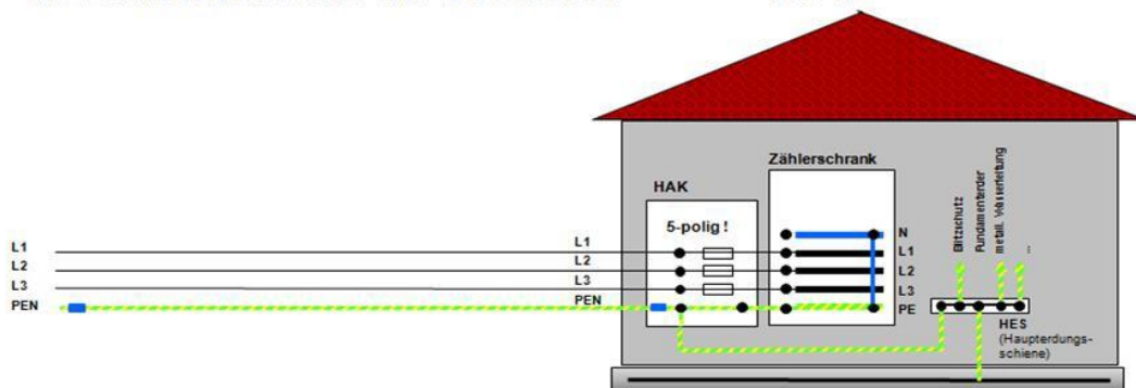
Abb. 18: Anschlussvariante bei SWM zur Innenanschlusstechnik (beispielhafte Darstellung)
